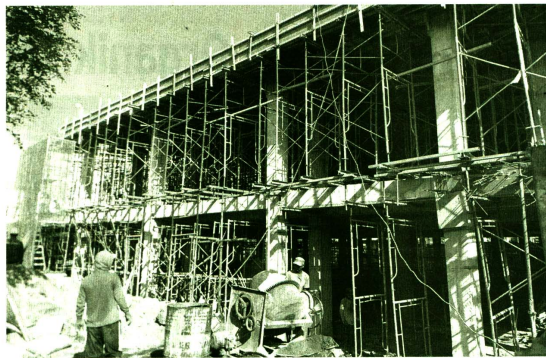
Suasana pengecoran lantai tiga dalam proyek pembangunan Pasar Sentul, seperti terlihat, Senin (14/8). Saat ini progres pembangunan Pasar Sentul baru mencapai 25%.
